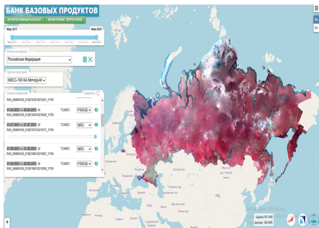
Рис. 3. Интерфейс доступа к бесшовному сплошному покрытию на основе данных с КА типа «Метеор-М», аппаратура КМСС-100, БИК-красный-зеленый, разрешение 60 м, территория РФ
